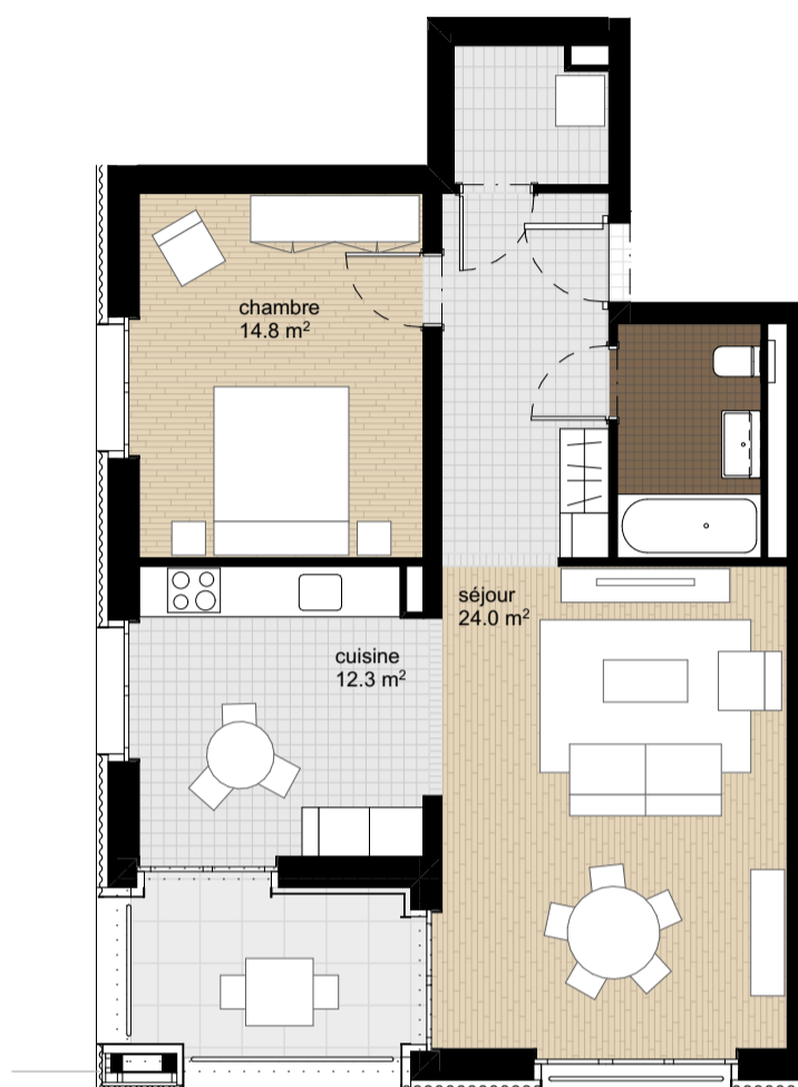
Plan de l'appartement, éch. 1:100
